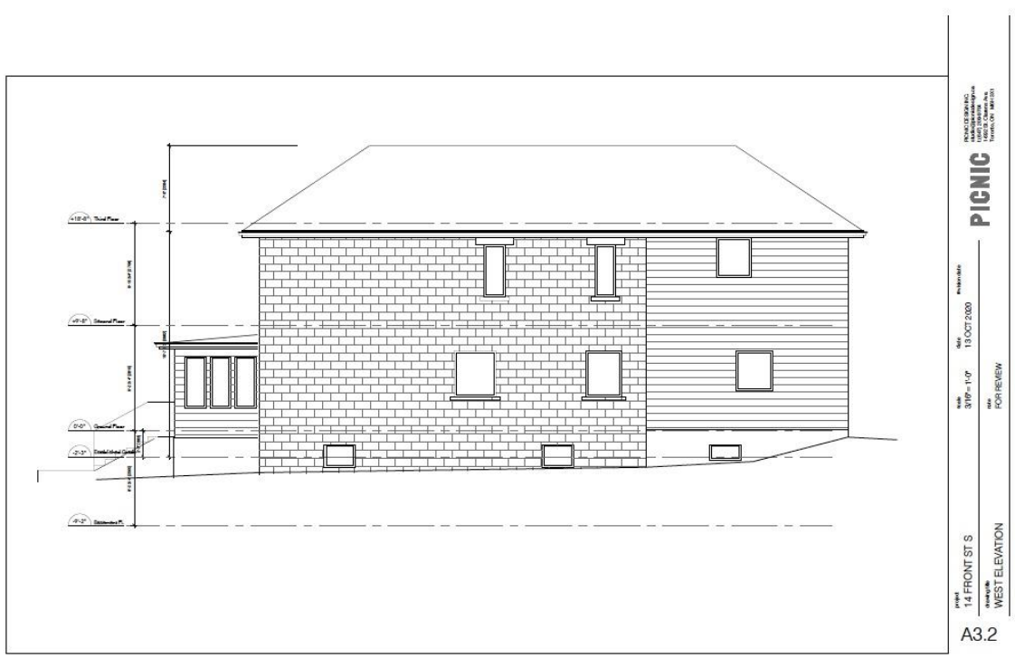
Existing West Elevation n.t.s.
