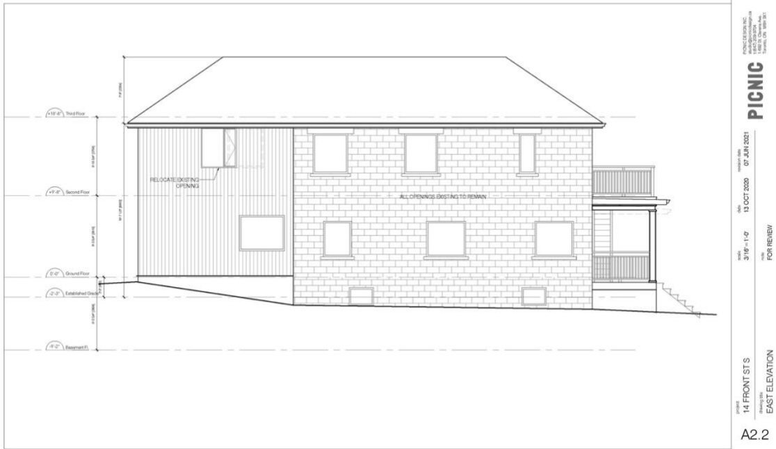
East Elevation n.t.s
