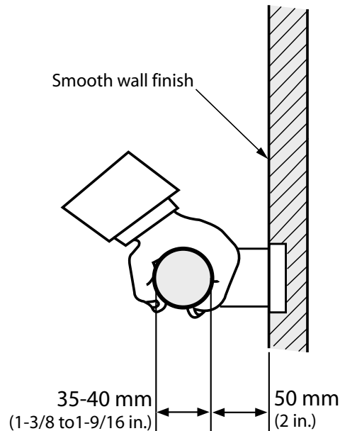
Figure 4.2.10.1 Grab Bar
