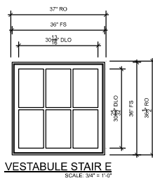
VESTIBULE STAIR E SCALE: 3/4" = 1'-0"
