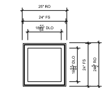
24X24 SQ STAIRS TOP SCALE: 3/4" = 1'-0"
